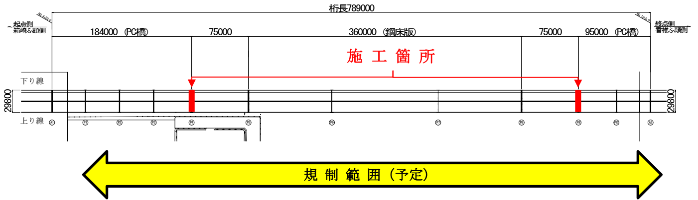
(平面図)
